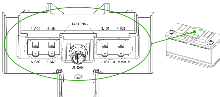
Abbildung 4. Signalschnittstellen
