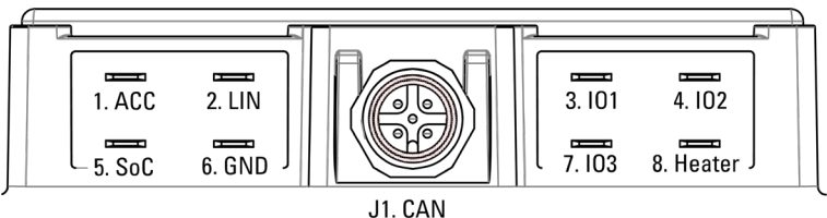
Abbildung 6. FASTON-Anschlüsse. Hinweis: Die FASTON-Anschlüsse sind auch auf der Innenseite des Schutzdeckels abgebildet.
