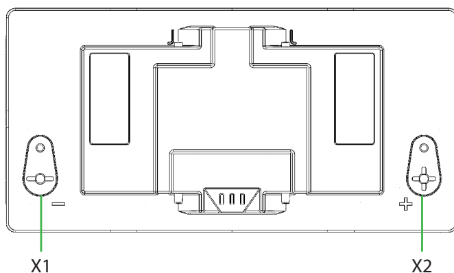
Abbildung 2. Batterieklammern
